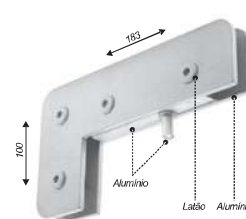
Fação simples para bandeira e fixo
