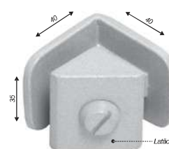
Suporte de centro para união de 2 vidros a 90°
