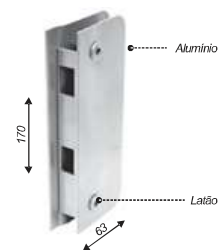
Contra fechadura V/V p/ 1510.MAC
