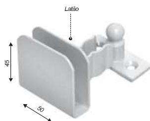
Fixador de porta rodapé/piso
