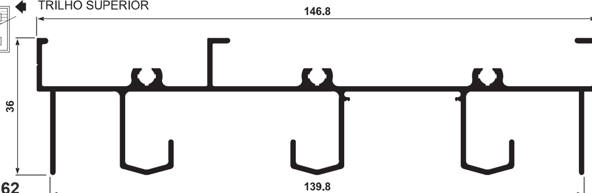
TRILHO SUPERIOR
