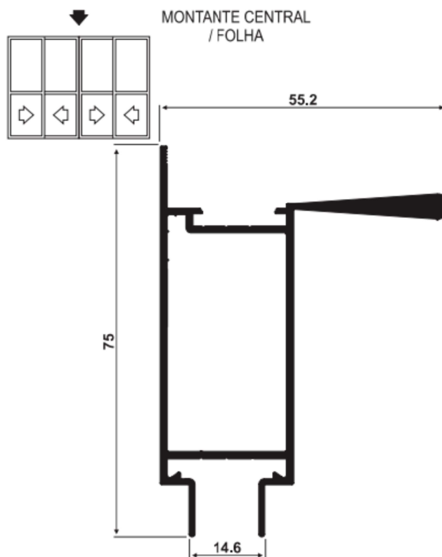
SU-281 1,029 Kg/m
