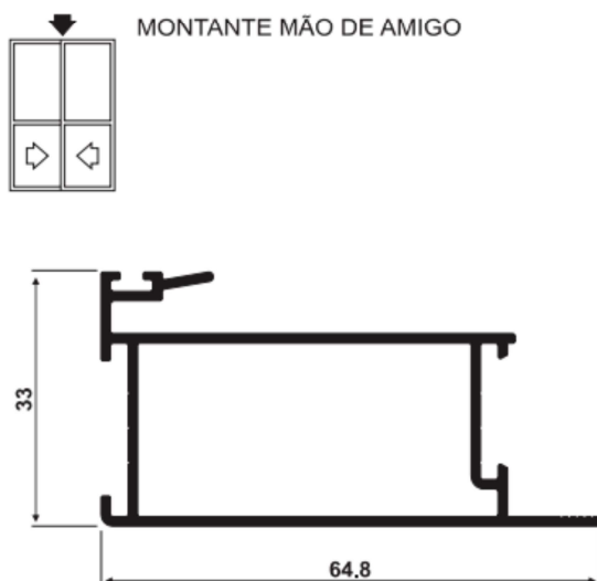
SU-280 0,969 Kg/m
