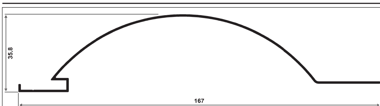
LB-038 0,693 kg/m
