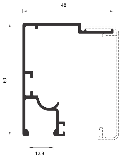
VT-59 0,621 kg/mt
