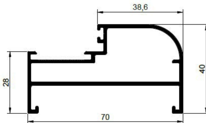
30-035 0,949 kg/m
