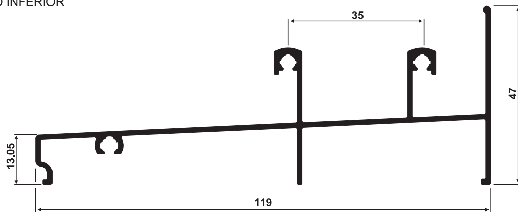
← MARCO INFERIOR
