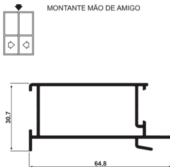
SU-281 1,029 Kg/m
