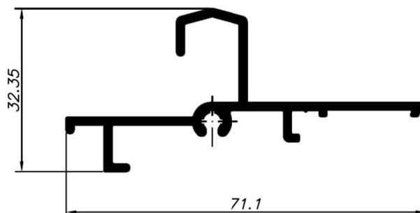
LG-575 0,595 KG/M
