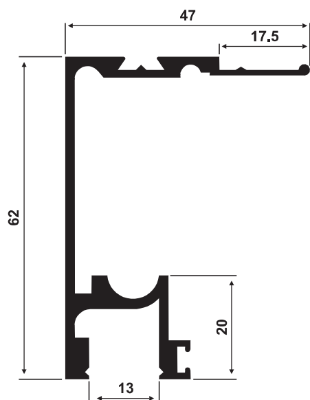
VT-01 0,990 Kg/m
