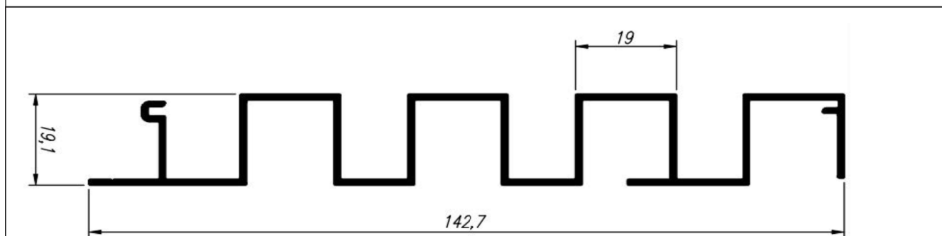
LB-005 0,446 kg/mt
