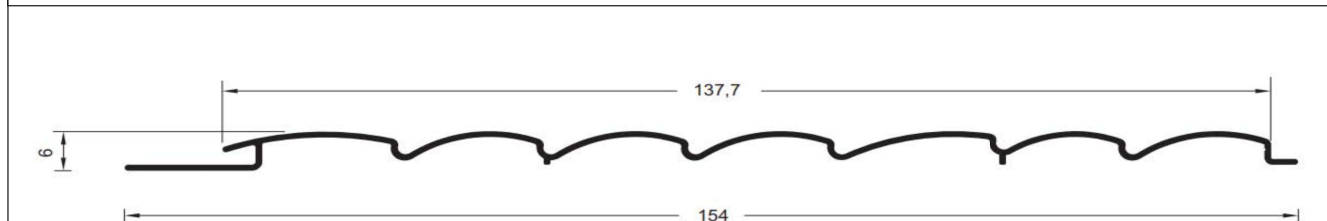
LB-050 0,529 kg/mt
