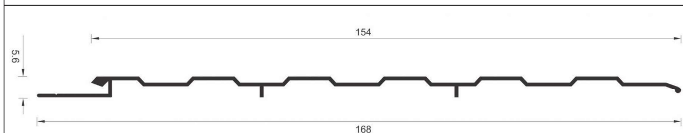
LB-038 0,693 kg/m
