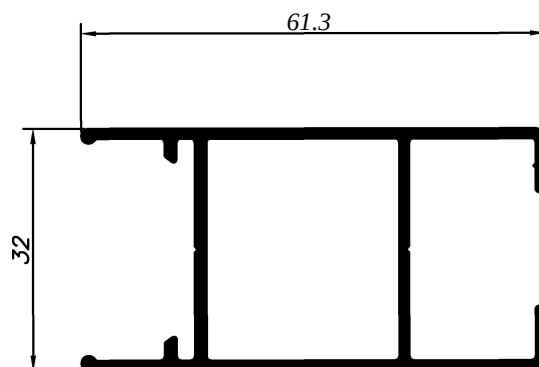
LG-632 0,789 Kg/m
