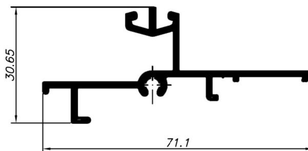
LG-573 0,612 KG/M
