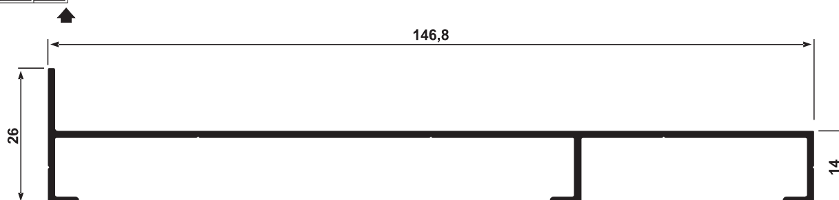
LG158 0,849 kg/m
