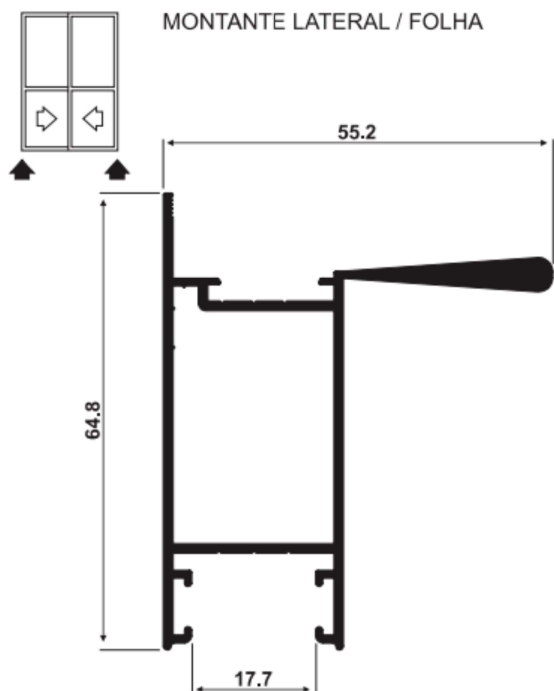
SU-280 0,969 Kg/m
