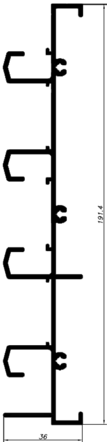
LG-570 1,976 KG/M
