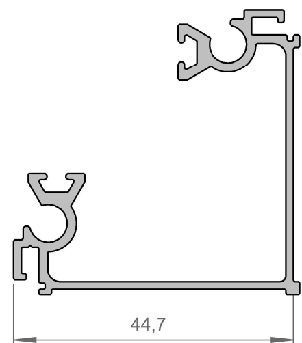
AT-269 - 0,623 kg/mt
