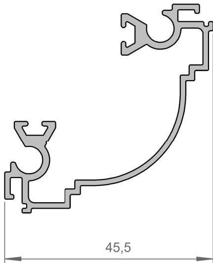
AT-273 - 0,590 kg/mt
