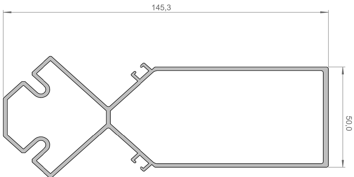
AT-236 - 2,343 kg/mt Coluna Ângulo 90 °
