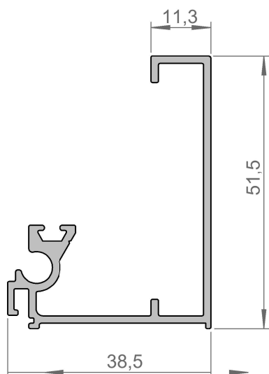
AT-228 - 0,572 kg/mt
