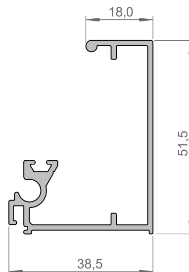
AT-232 - 0,607 kg/mt
