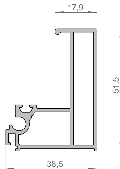
AT-230 - 0,813 kg/mt
