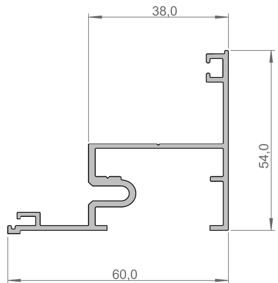
AT-294 - 0,774 kg/mt
