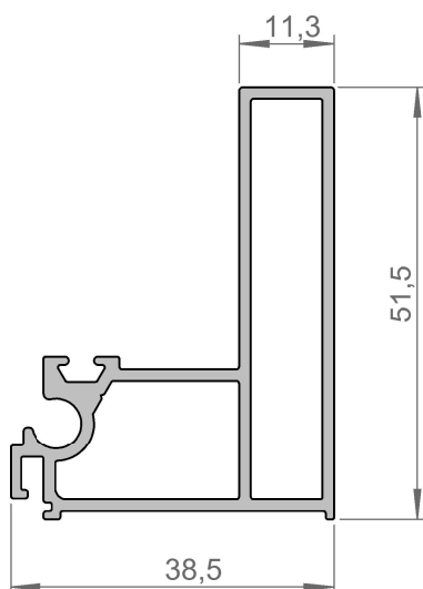
AT-245 - 0,784 kg/mt
