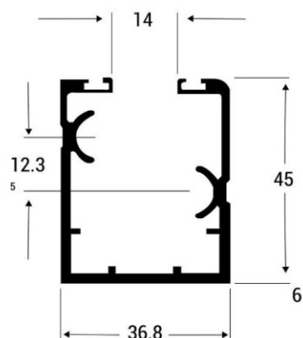
Trilho inferior
