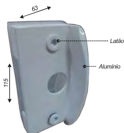
Fechadura para portas de correr com furação
