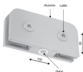
Dobradiça pino para basculante 50x100mm
