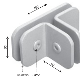
Suporte para união de 3 vidros (sem núcleo)
