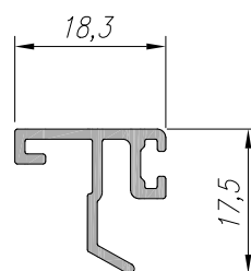
ES-1213 ACABAMENTO 0,183 kg/m
