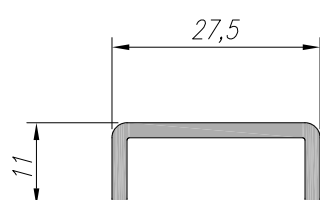
ES-767 CORRIMÃO 0,240 kg/m
