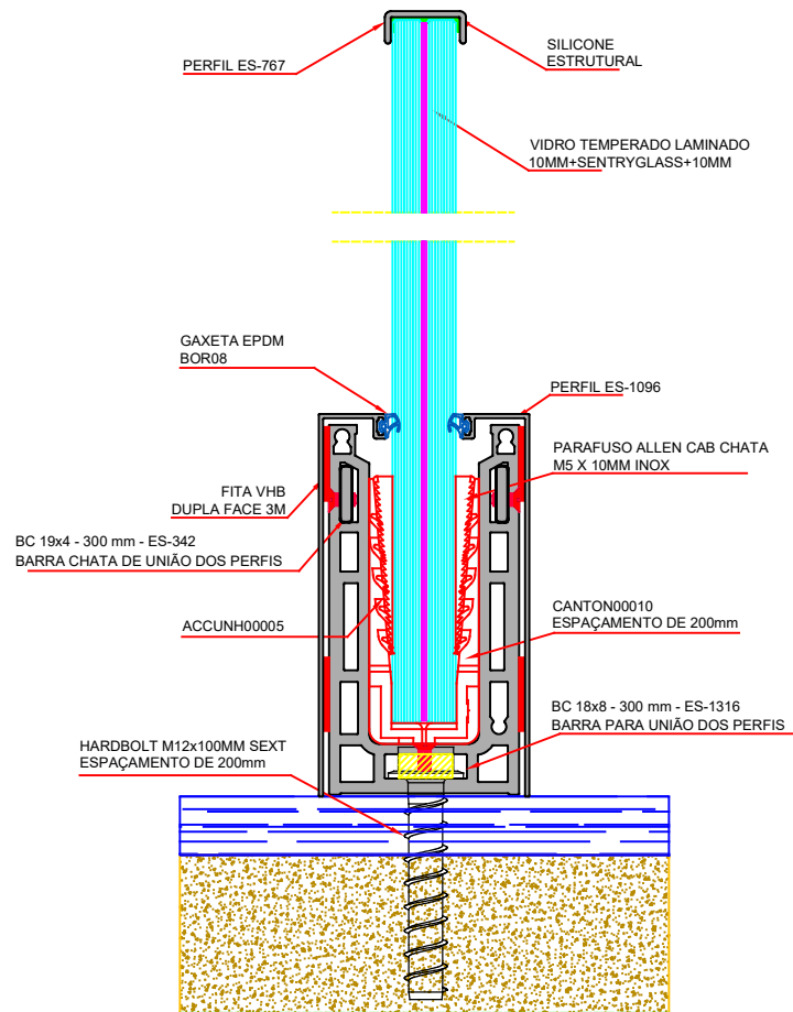
Guarda Corpo Auto Portante - Instalação sobre laje
