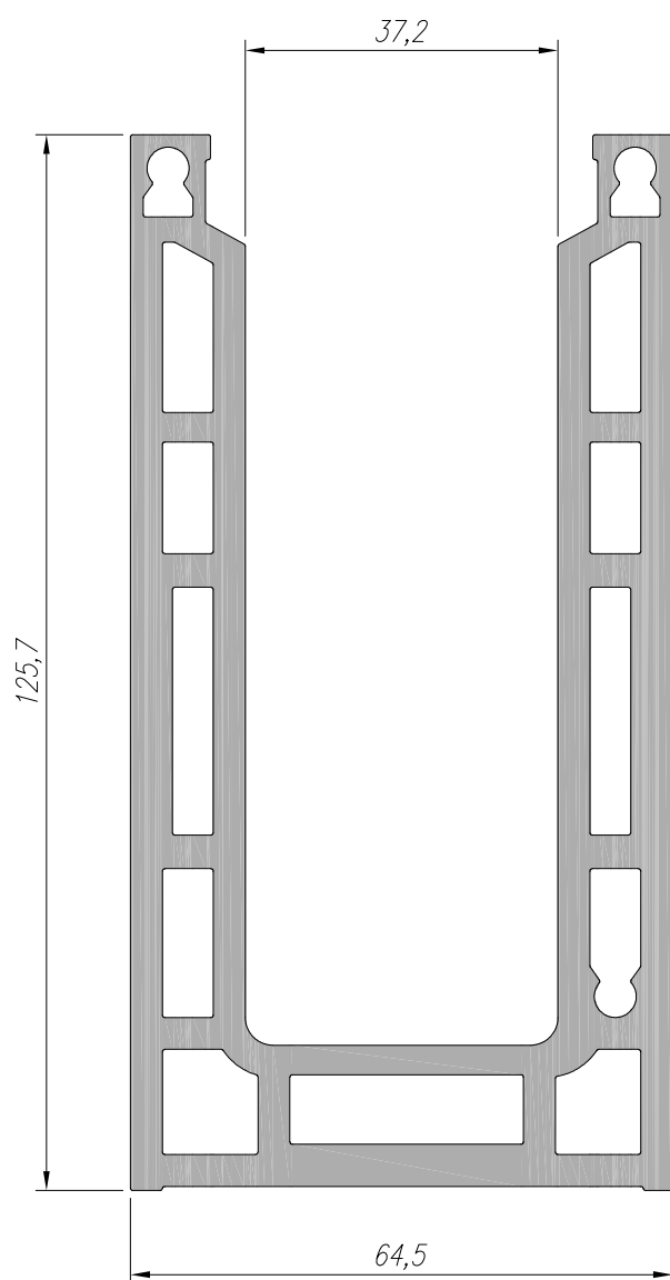
ES-768 PERFIL ESTRUTURAL 6,775 kg/m
