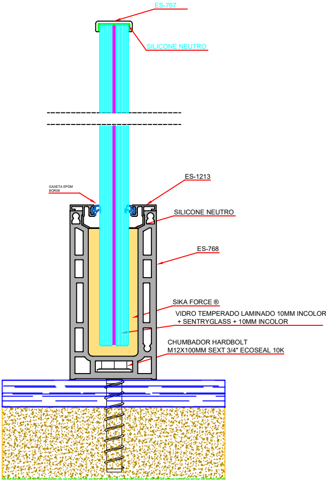
Corte A
