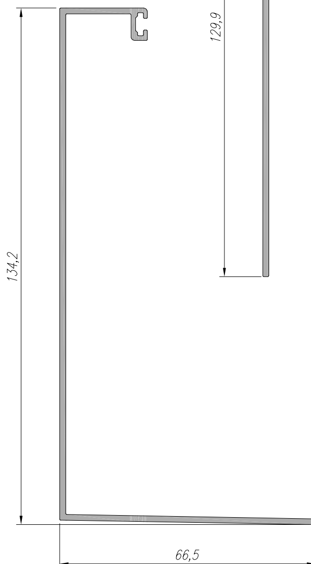
ES-1214 ACABAMENTO 0,967 kg/m
