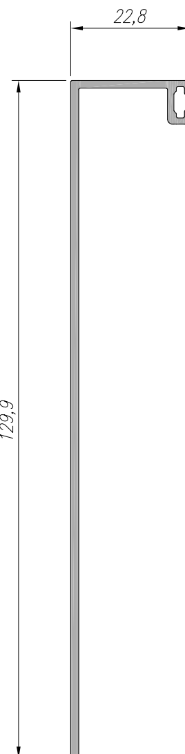
ES-1096 ACABAMENTO 0,654 kg/m
