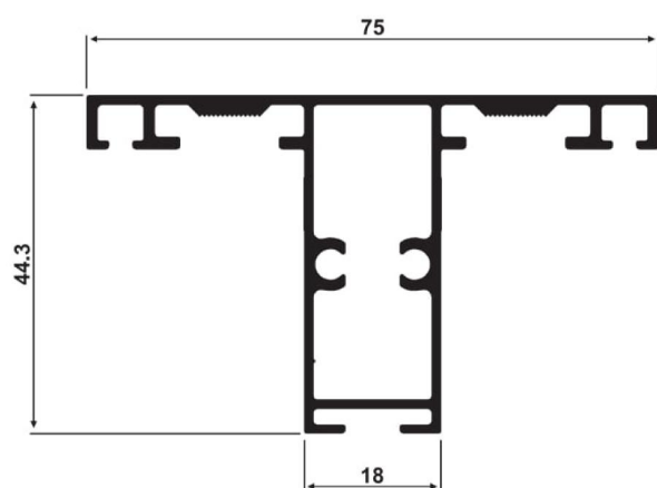
FC-231 FC-231 0,996 kg/m
