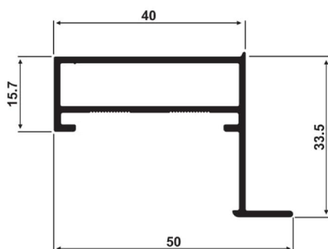
FC-228 FC-228 0,554 kg/m
