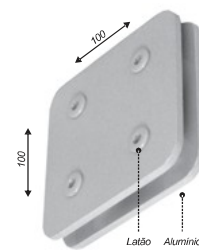
Suporte sem núcleo para união de 4 vidros
