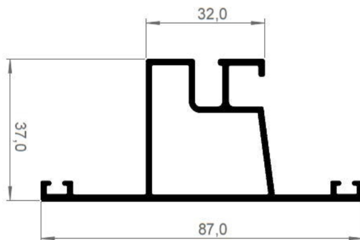
AT-233 - 0,886 kg/mt Travessa Horizontal
