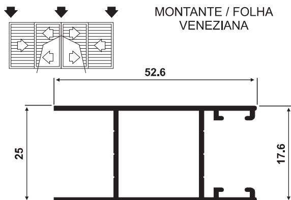
SU-068 0,509 Kg/m
