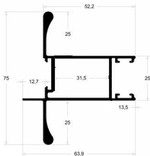
SU-299 0,966 kg/m
