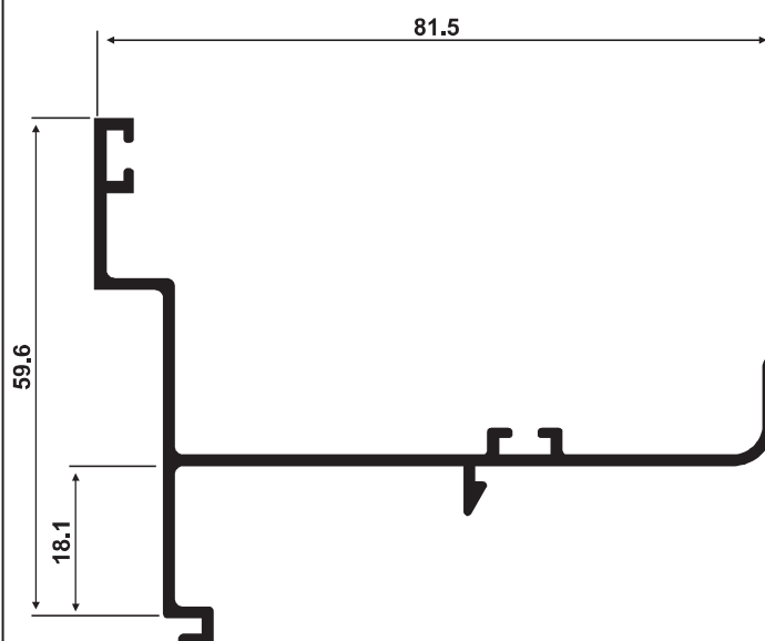
FC-226 0,713 kg/m
