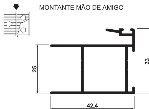
SU-070 0,494 Kg/m
