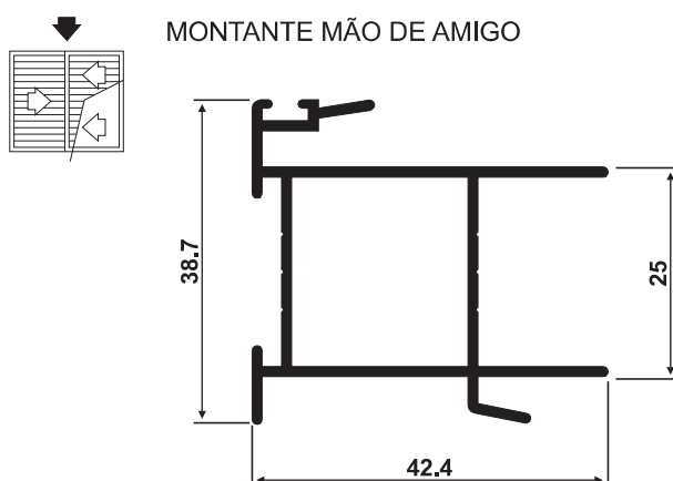
SU-069 0,547 Kg/m
