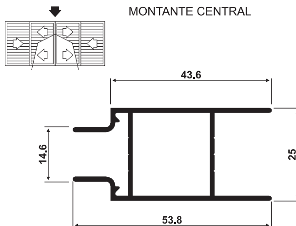
SU-191 0,514 Kg/m
