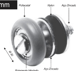
Roldana para porta de correr (rolamento importado)
