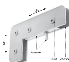
Facão simples para bandeira e fixo
