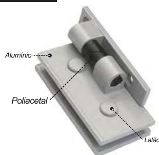
Dobradiça automática para box
