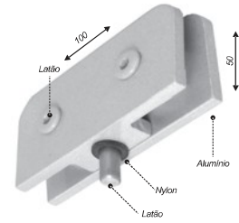
Dobradiça pino para basculante 50x100mm
