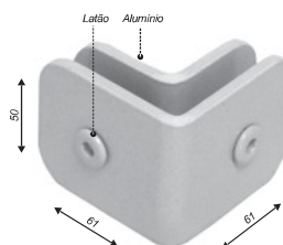
Suporte central para união de 2 vidros a 90°
