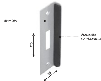
Contra Fechadura V/A p/ 3530 e 3532
