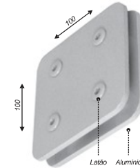
Suporte sem núcleo para união de 4 vidros
