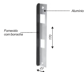
Contra fechadura VIA p/ 1510.MAC
