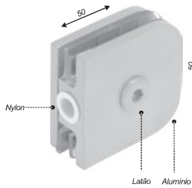
Dobradiça bucha para basculante 50x50mm
