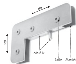
Fação simples para bandeira e fixo
