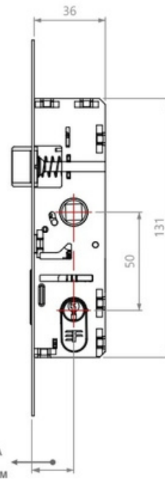
FECHADURA 3F PORTA DE GIRO C/MAÇ ESPECIAL
