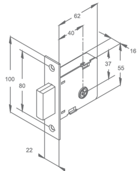
FECHADURA AUXILIAR INOX P/ ESQUADRIA L.30 FRA-1004
