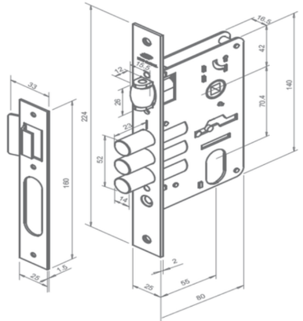
KIT FECHADU INOX ROLETE MULTIPONTO 70MM FRA-1007-IMAB
