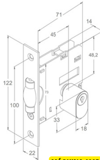
CROM. C/ROLETE PIVOTANTE LINHA 30 85MM STAM FRA826S
