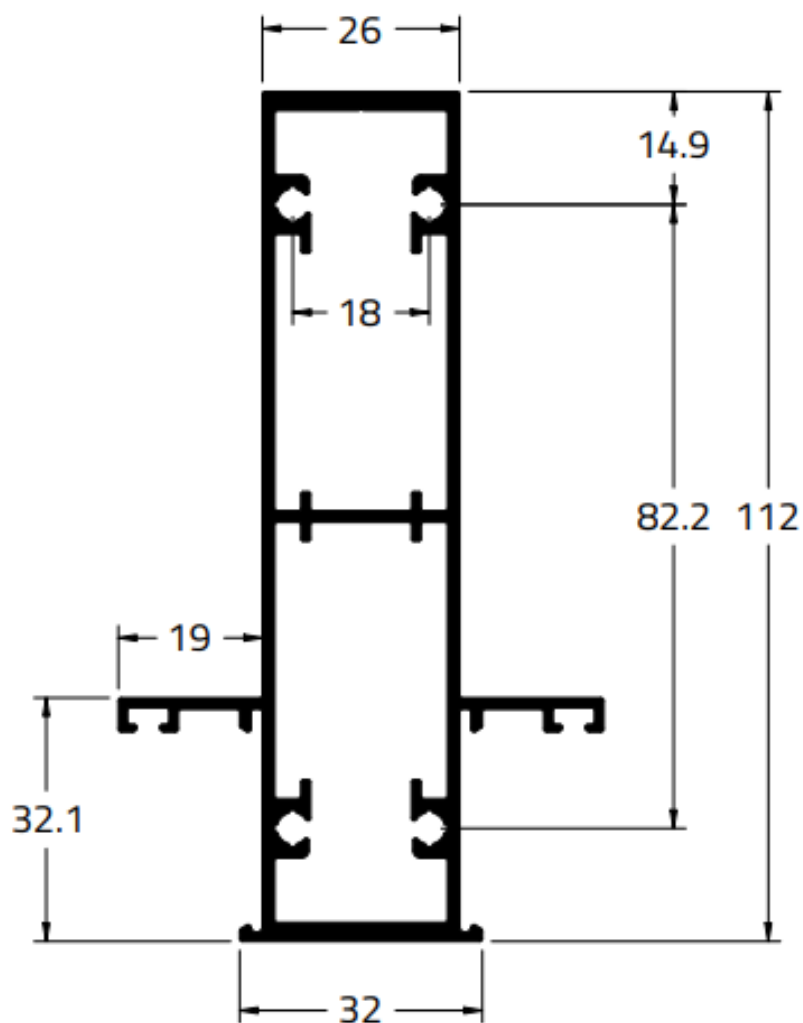
CHR-705 0,347 Kg/m
