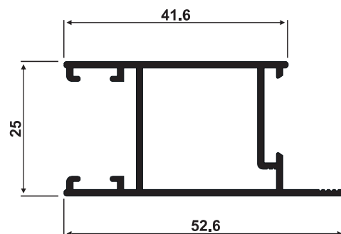
SU-039 0,506 Kg/m
