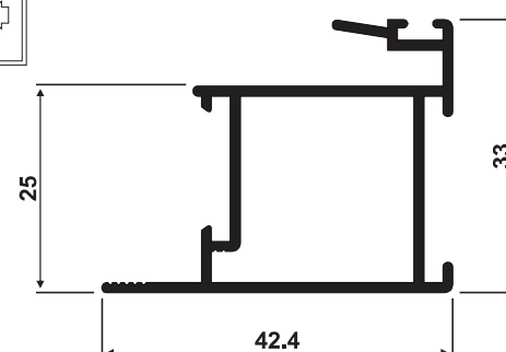
SU-041 0,485 Kg/m
