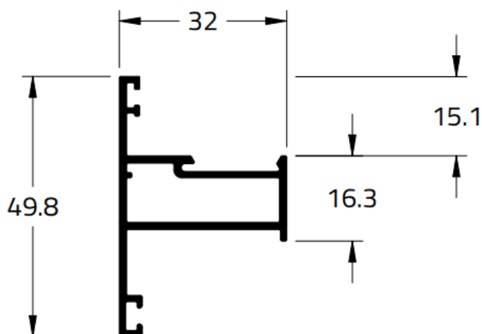
CHR-713 0,544 Kg/m
