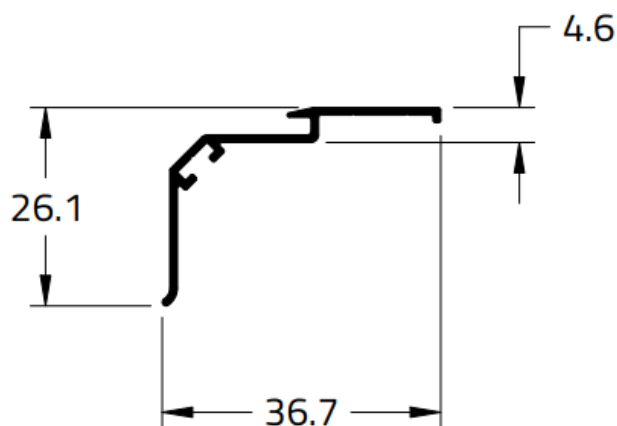
CHR-885 0,191 Kg/m
