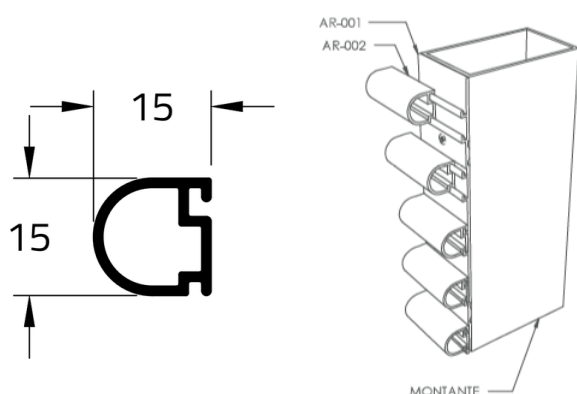
AR-002 0,186 kg/mt
