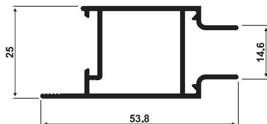
SU-192 0,498 Kg/m
