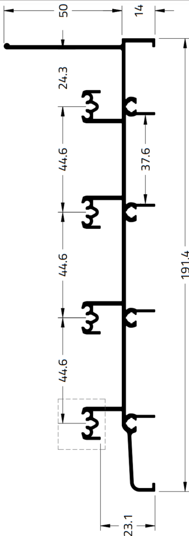
CHR-020 2,199 Kg/m
