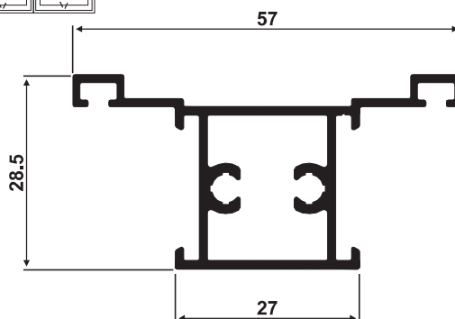
SU-086 0,581 Kg/m
