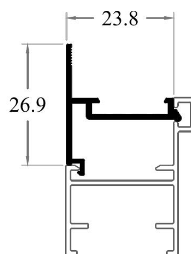
SU-292 0,214 kg/m
