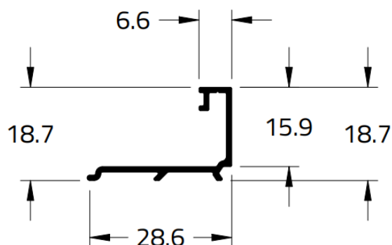
CHR-712 0,183 Kg/m
