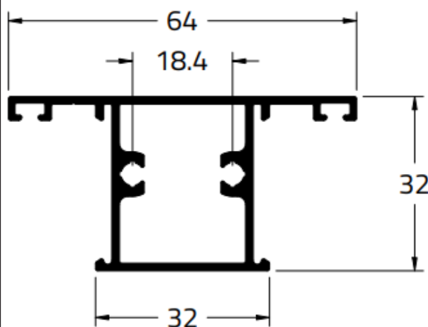
CHR-703 0,801 Kg/m
