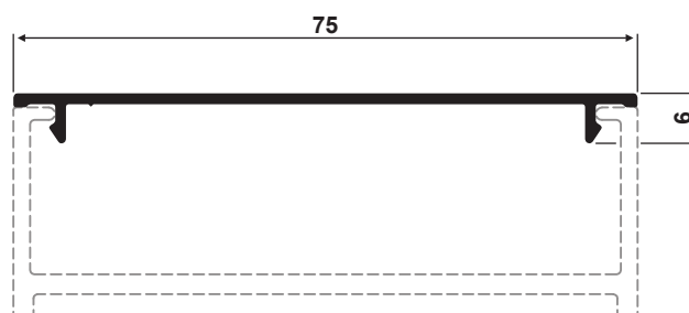
FC-234 0,316kg/m
