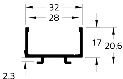
CHR-121 0,335 Kg/m
