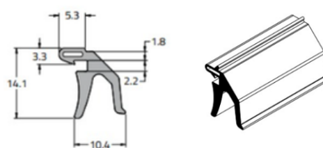
GUARNIÇÃO DE BORRACHA PSC003
