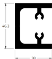
PRESILHA PARA TRAVESSA 49MM GPC08-200
