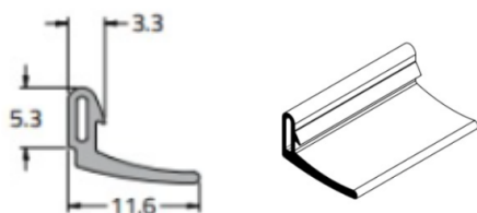
GUARNIÇÃO DE BORRACHA PSC002
