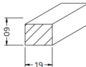
GUARNIÇÃO ESP ADESIVA 19 X 09 GUA1909
