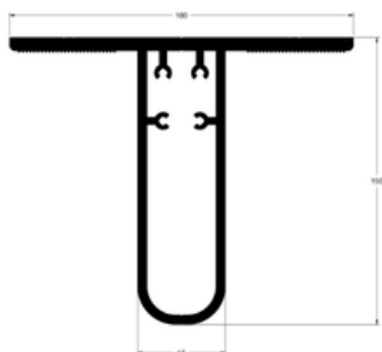
ANCORAGEM PARA MONTANTE 100,7MM GPC07-135
