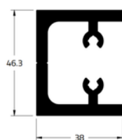
PRESILHA PARA TRAVESSA 102MM GPC08-135
