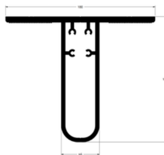
ANCORAGEM PARA MONTANTE 165,7MM GPC07-200
