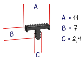
GUARNIÇÃO BORRACHA GUA504-T PARA FACHADA GUA504-T
