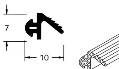
GUARNIÇÃO GUA239 GUAC239
