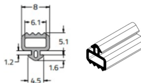
GUARNIÇÃO DE BORRACHA PSC001
