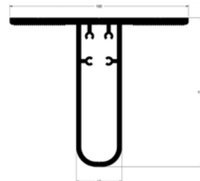
ANCORAGEM PARA MONTANTE 65,7MM GPC07-100
