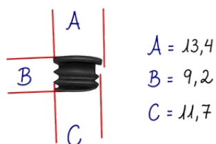
GUARNIÇÃO BORRACHA GUA016 PARA FACHADA GUA016
