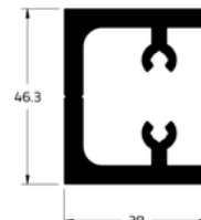
PRESILHA PARA TRAVESSA 67MM GPC08-100
