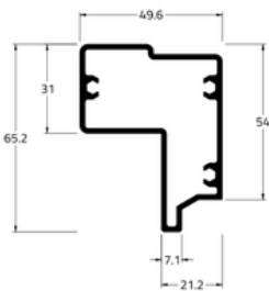
LUVA DO MARCO PARA COLUMNA PS-317 LUV339
