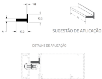
CALÇO DE APOIO PARA VIDRO 50MM GPC009-050
