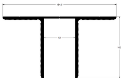
ANCORAGEM COLUNA CENTRAL GPC017
