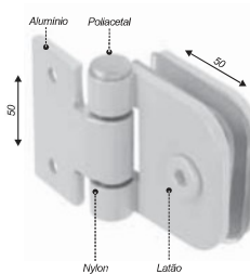
Dobradiça simples pequena para janela
