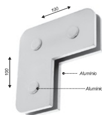
SUPORTE PARA UNIAO DE 3 VIDROS
