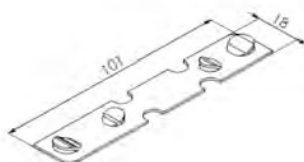
CON 063 CONTRA MARCO CN 063 E CN 200
