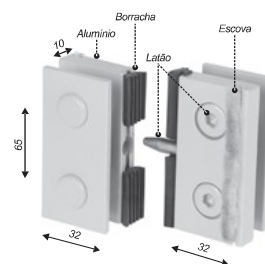
Mini conjunto mão de amigo para sistema 1030
