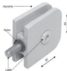
Dobradiça pino para basculante
