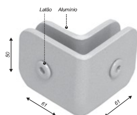
Suporte central para união de 2 vidros a 90°
