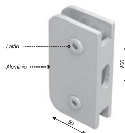
Contra-fechadura para 1520/1550
