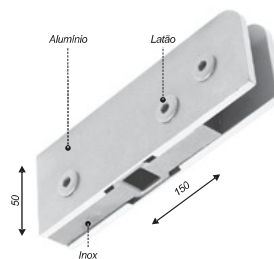
Dobradiça inferior com miolo inox para mola para porta até 1000mm*
