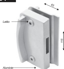
Contra Fechadura V/V p/ 3530
