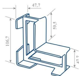
CANTO 50 X 50 PARA PERFIL TQ-047
