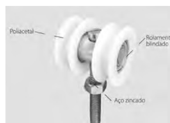
Roldana Dupla p/ Trilho
