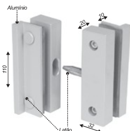
Conjunto mão de amigo para portas de correr com sistema deslizante
