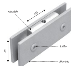
Suporte de canto com rosca para roldana 1150
