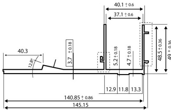
Prolongador
