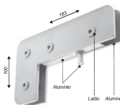
Facão simples para bandeira e fixo
