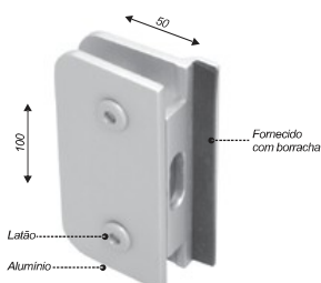
Contra-fechadura V/V com batente para 1520
