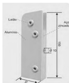
Dobradiça inferior
