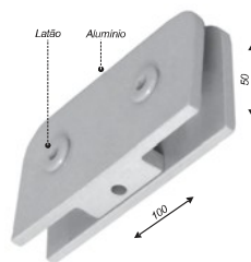
Suporte para união de 2 vidros
