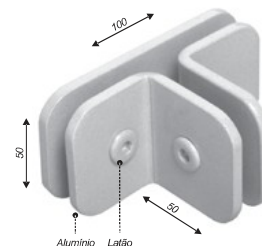
Suporte para união de 3 vidros (sem núcleo)
