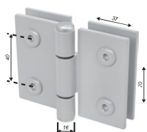
Dobradiça MAXIM-AR V/V 40mm entre furos
