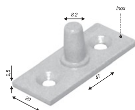
Pivô em inox para 1101, 1230 e 1231
