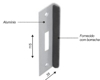
Contra Fechadura V/A p/ 3530 e 3532
