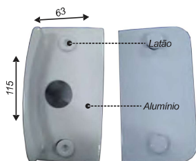
Fechadura p/ janela de correr (sem tambor e puxador externo)
