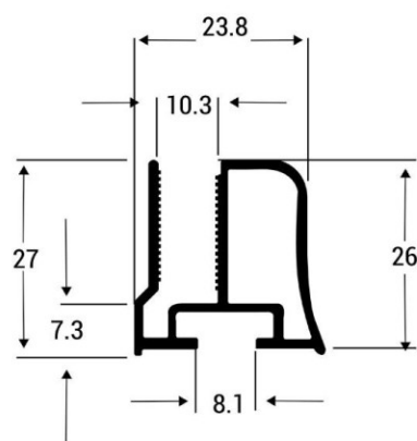
Perfil leito para vidros 10mm
