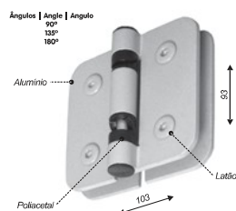
Dobradiça automática dupla Direita e Esquerda
