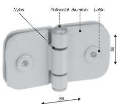
Dobradiça dupla pequena para janela
