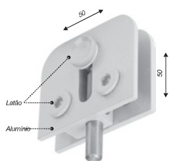
Trinco central para janela e porta de correr
