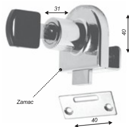
Fechadura de pressão com lingueta para rack
