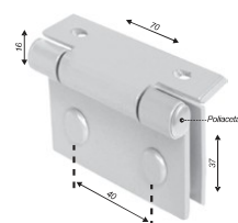
Dobradiça MAXIM-AR V/A 40mm entre furos
