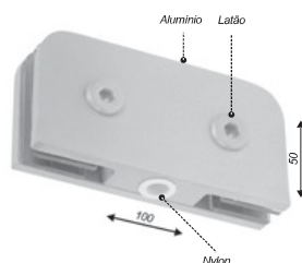
Dobradiça pino para basculante 50x100mm
