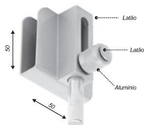
Trinco de pressão sem núcleo
