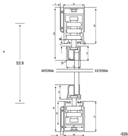
Kit montado
