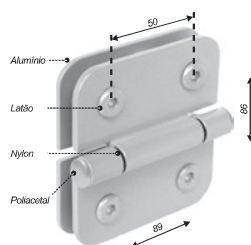
Dobradiça MAXIM-AR V/V (50mm entre furos)
