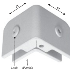
Suporte piso / Teto para união de 2 vidros a 90°
