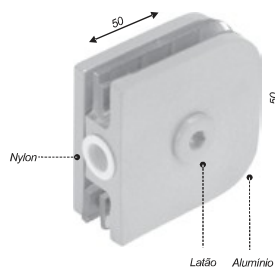
Dobradiça bucha para basculante 50x50mm
