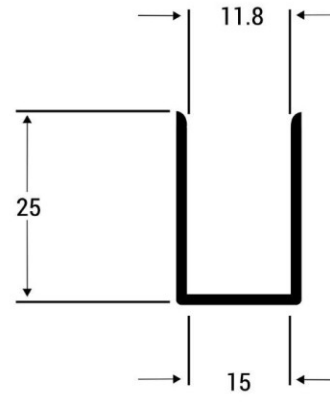
Perfil "u"
