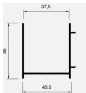
Perfil "U" de regulagem
