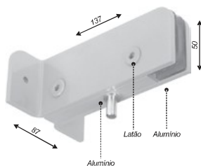
Suporte de bandeira para dobradiça 1101
