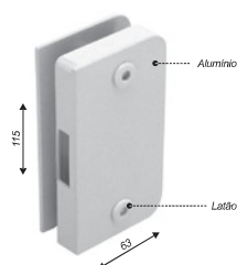
Contra Fechadura V/V para 1520X
