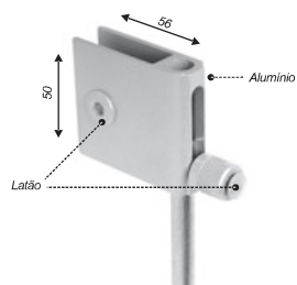
Trinco para janela de correr
