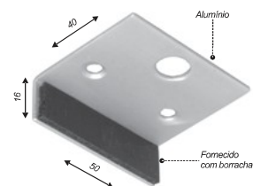
Batedeira para trinco de basculante
