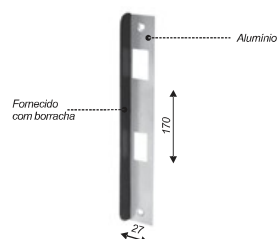
Contra fechadura V/A p/ 1510.MAC
