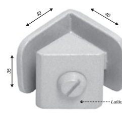
Suporte de centro para união de 2 vidros a 90°
