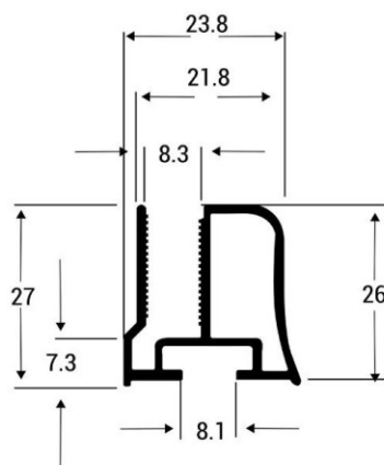
Perfil leito para vidros 8mm
