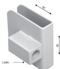
Contratrinco de pressão para 1800C
