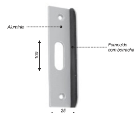
Batedeira em alvenaria para 1520
