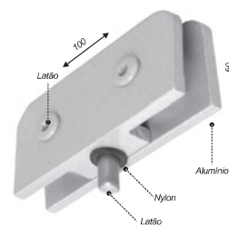
Dobradiça pino para basculante 50x100mm
